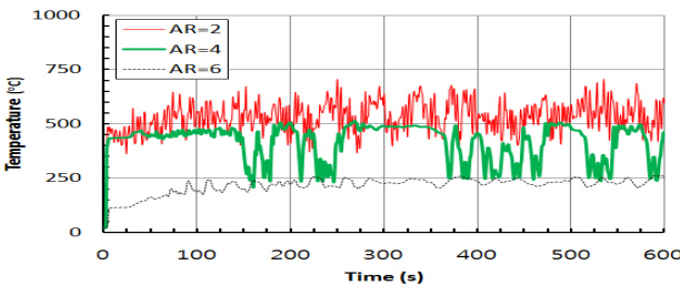
(d) 2 [MW] in enclosure L
