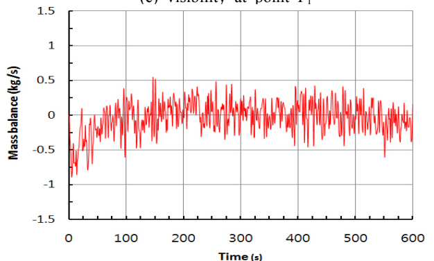
(d) mass balance through doors
